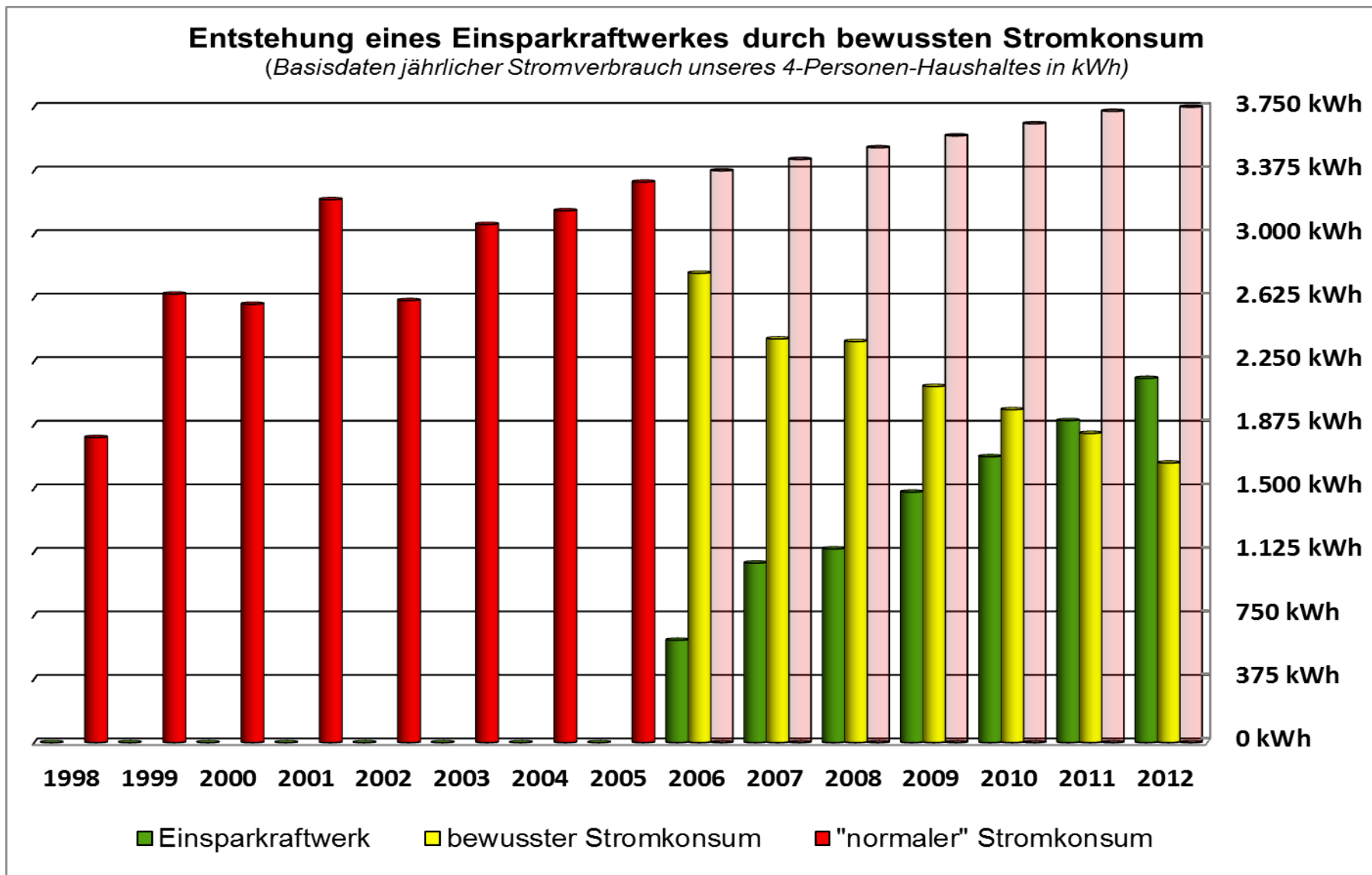
Abb. 9: Entstehung und Entwicklung eines Einsparkraftwerkes
